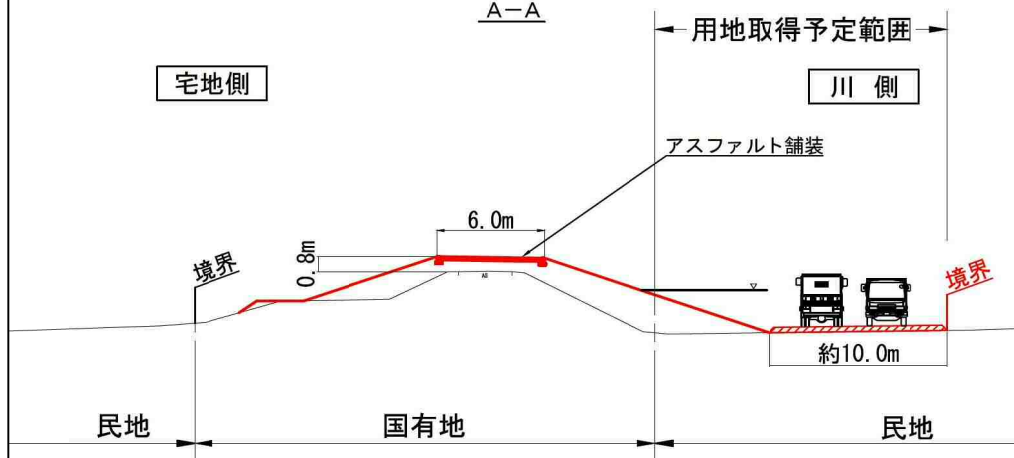
標準断面図 A-A
