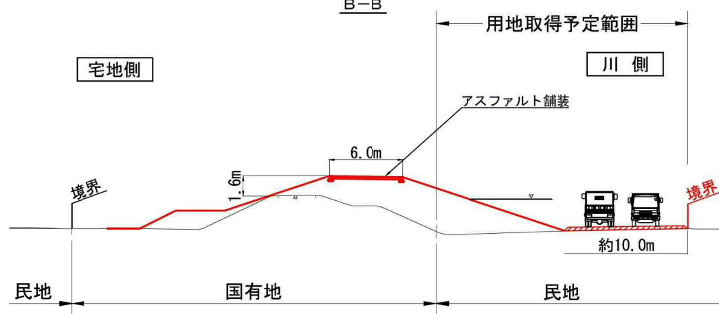
標準断面図 B-B
