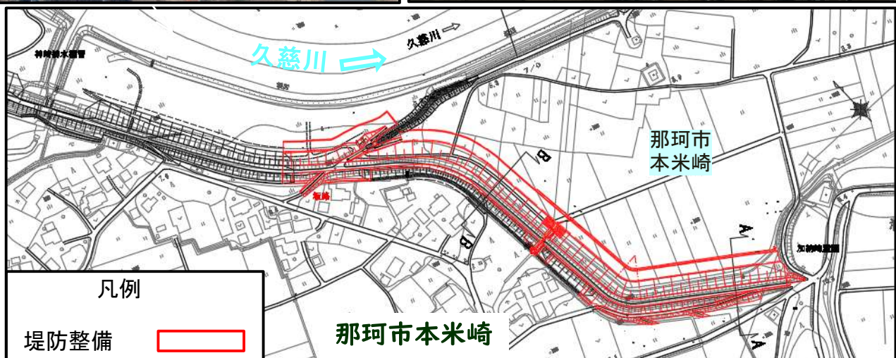
▲ 堤防整備平面図
