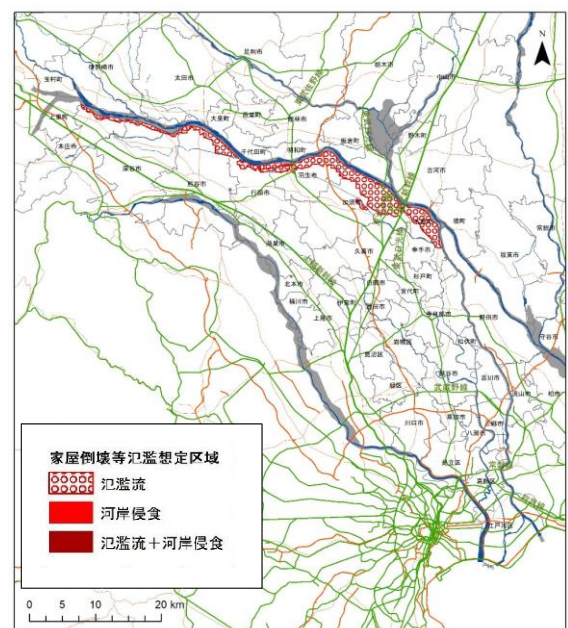
家屋倒壊等氾濫想定区域(氾濫流、河岸侵食)
