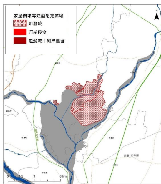
家屋倒壊等氾濫想定区域(氾濫流、河岸侵食) (想定最大規模)
