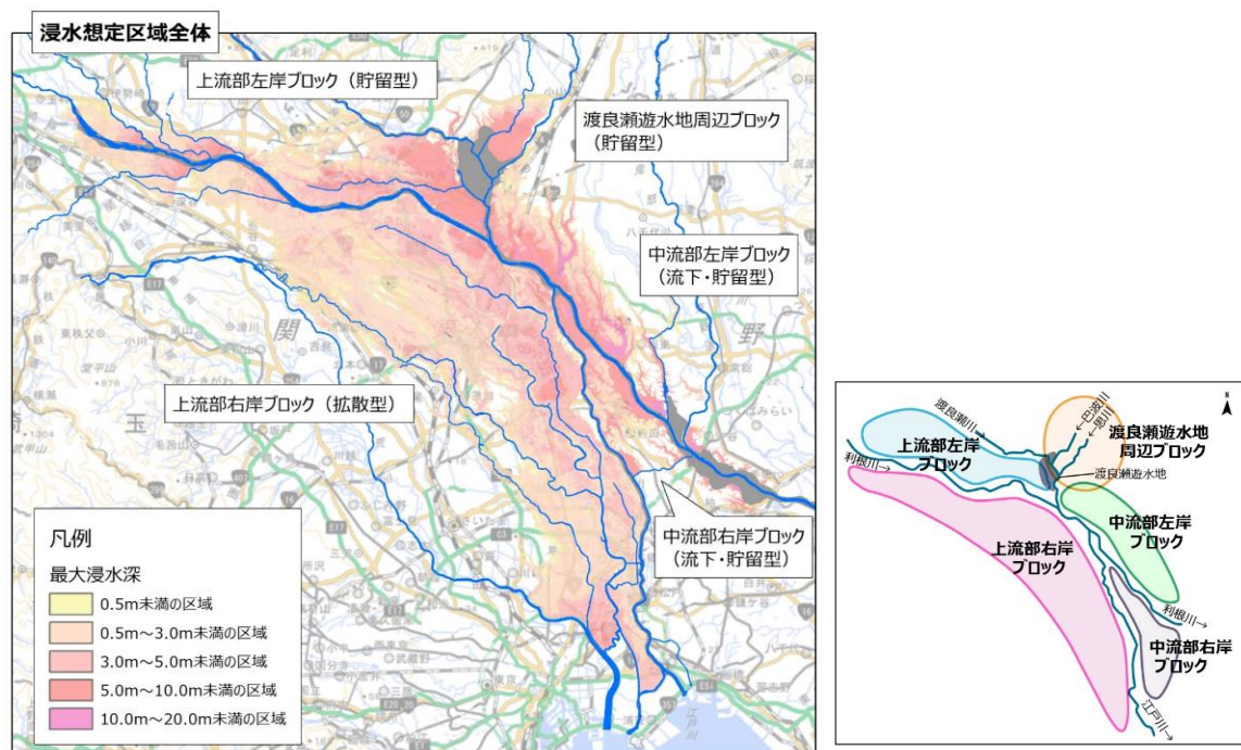
図 8 氾濫特性からみた利根川上流域の氾濫ブロック
