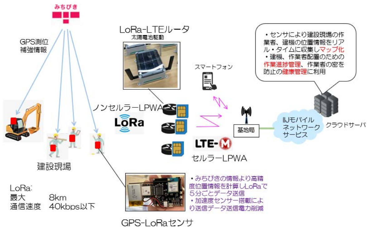
建設工事現場での測位データ収集ネットワーク展開構成と収集データの解析システム
