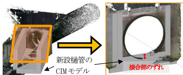
図 1-2 統合モデルでの接合部確認
