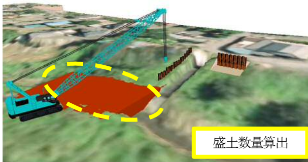
図5-1 重機及び施工数量の算出
