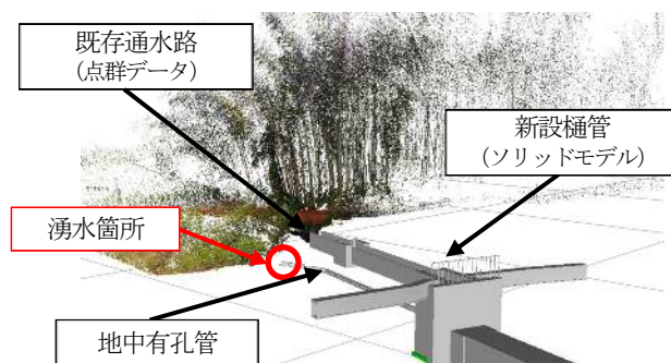
図 1-1 新設樋管と既存通路の接続部
