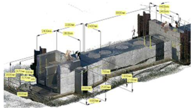
図3-2 取得した構造物の点群
