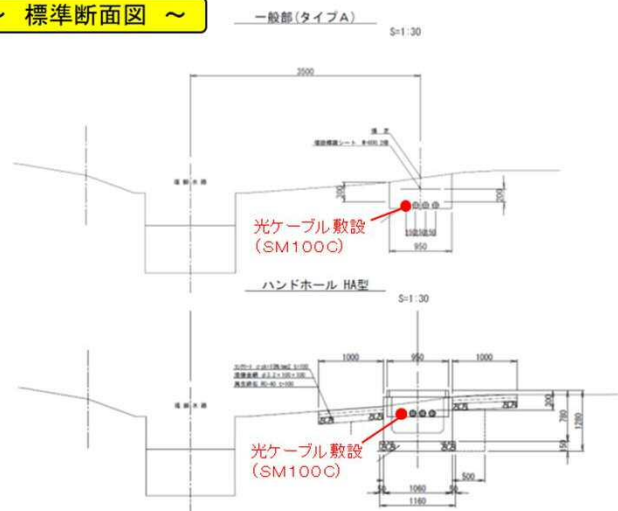
～ 標準断面図 ～
