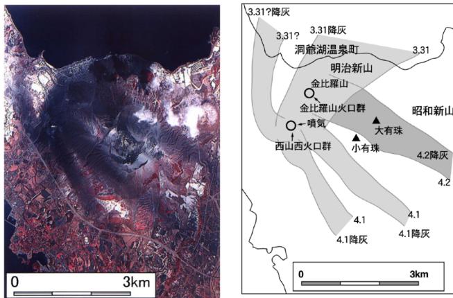
図 3-3 ASTER/VNIR 画像による降灰域の判読事例(2000 年 4 月 3 日の有珠山)
