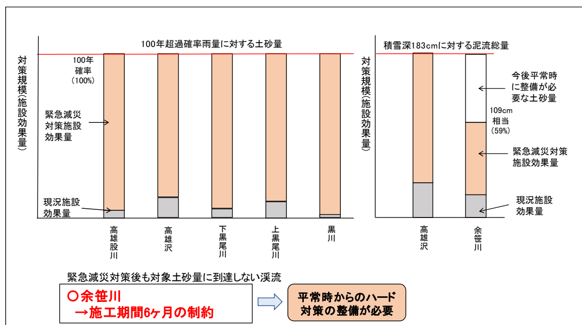
図 5-18 平常時からハード対策の整備が必要な溪流
