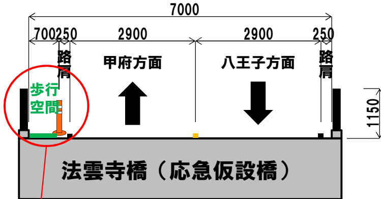
【現況断面図】 A-A断面
