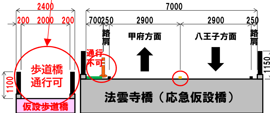
【計画断面図】 A-A断面
