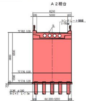
下部工正面図 S=1:100
