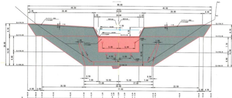
本堤正面図
