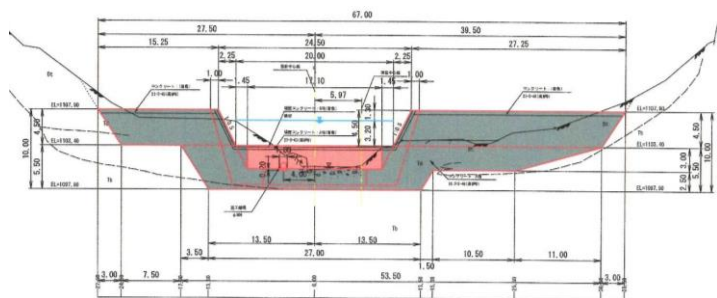
副堤正面図
