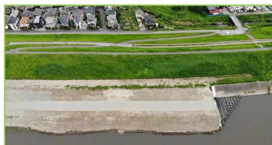
H30三輪野山地区低水護岸工事 完成写真
