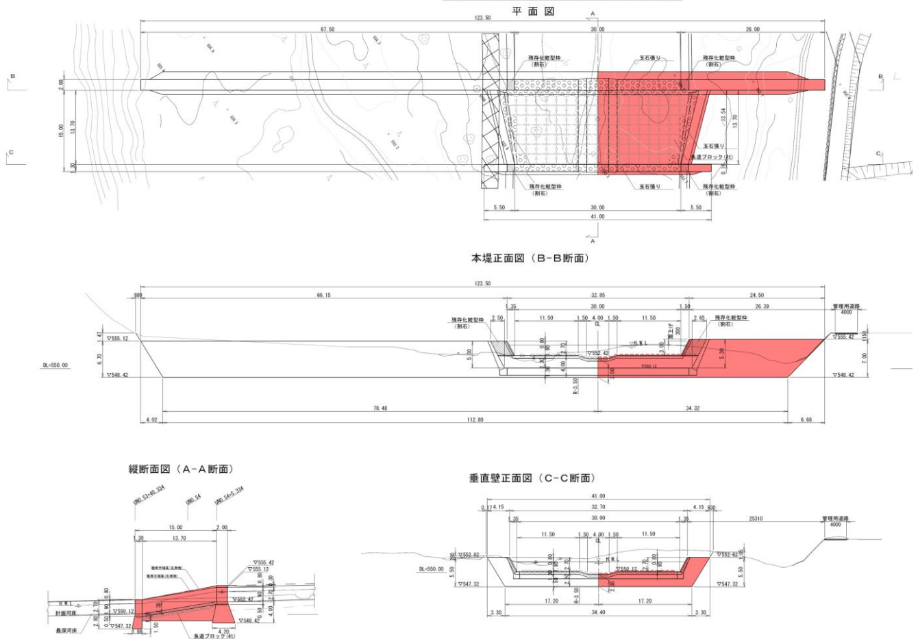
第二床固工一般図 S=1:300
