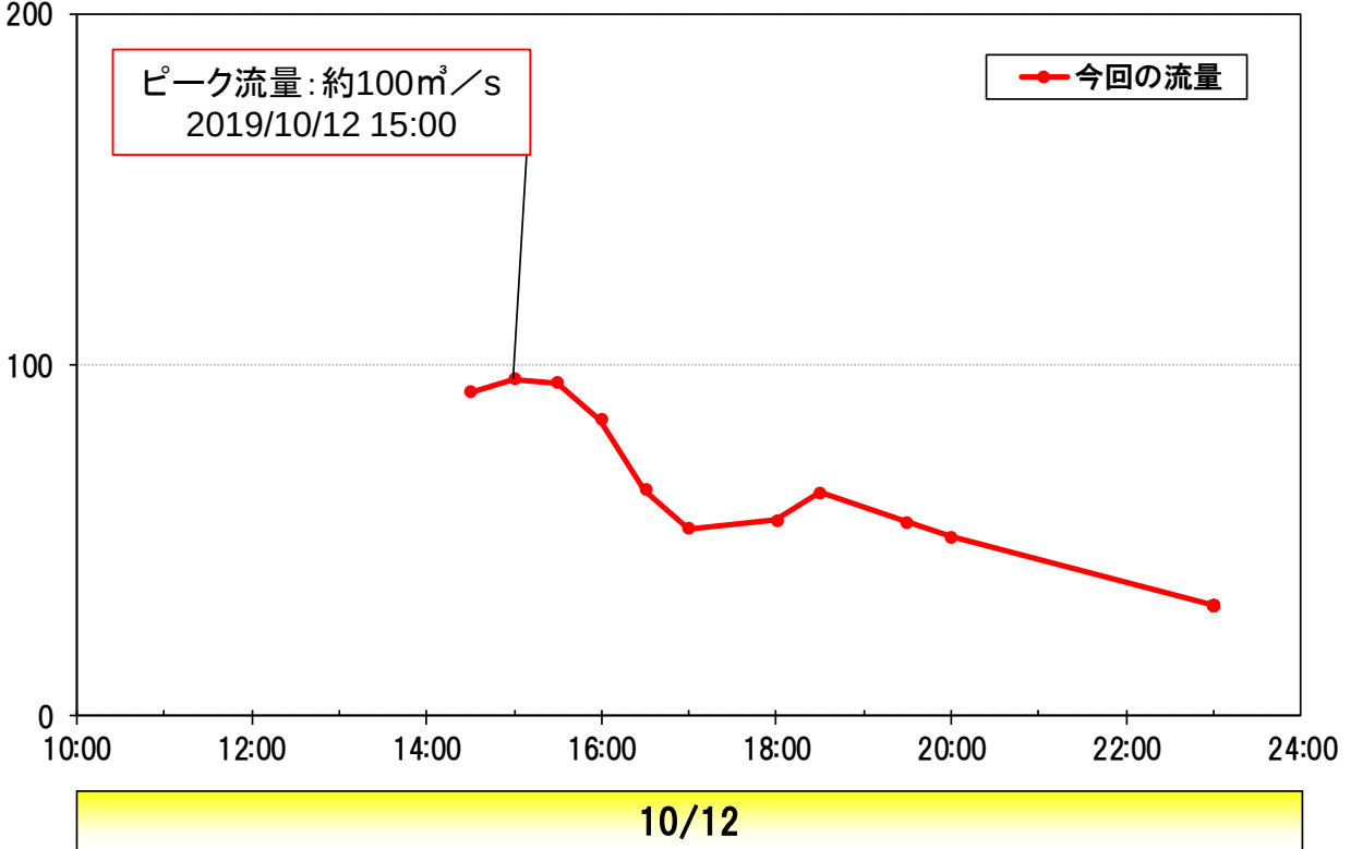
流量( \text{m}^3/\text{s} ) 高田橋流量観測所(早淵川1.4km 神奈川県横浜市港北区新吉田町)
