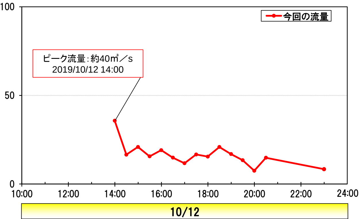
流量( \text{m}^3/\text{s} ) 鳥山流量観測所(鳥山川1.4km 神奈川県横浜市港北区鳥山町)
