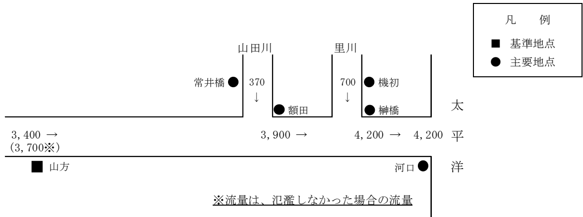
21 図 4-1 久慈川流量配分図 (単位 : m³/s)
