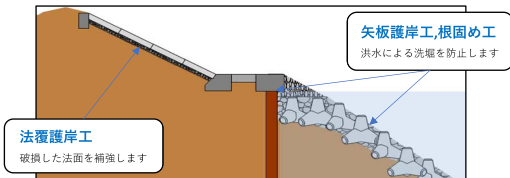
護岸整備イメージ
