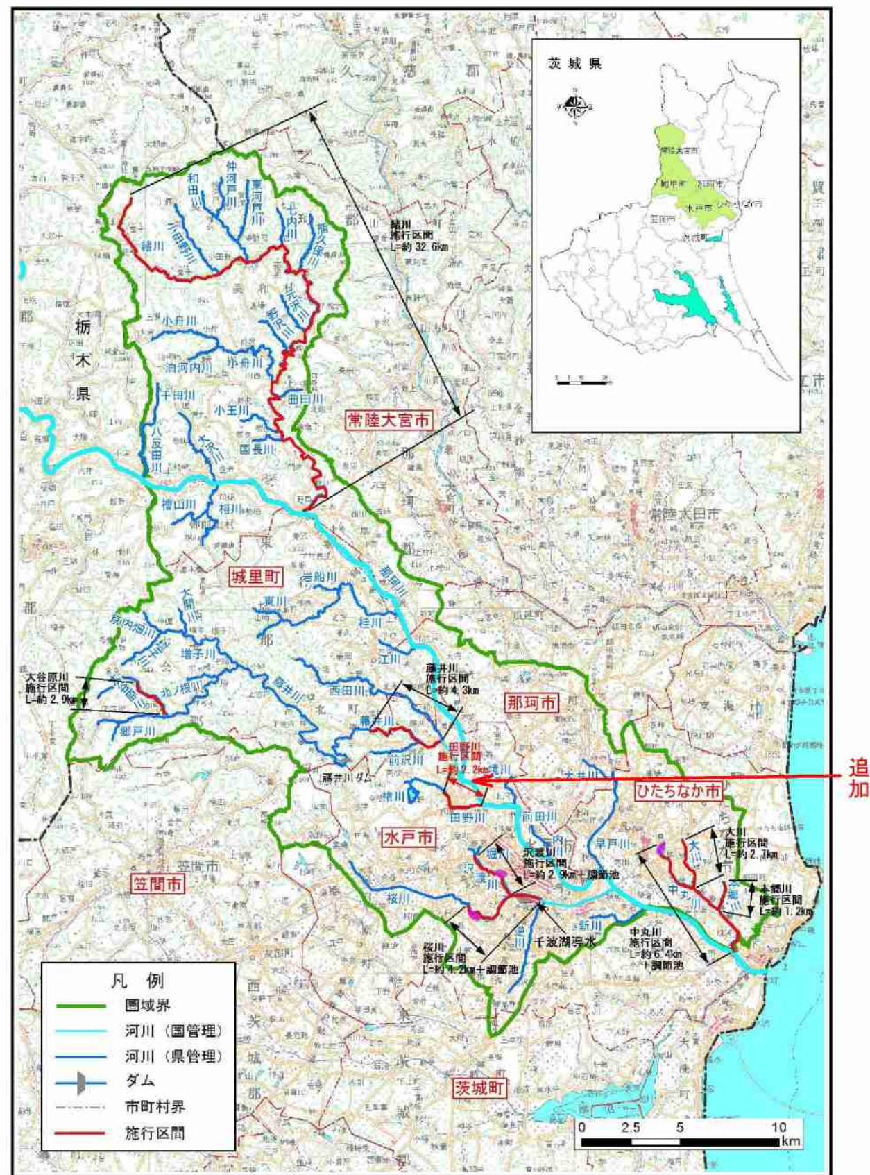
図 2-1 那珂川圏域河川整備の施行区間図
