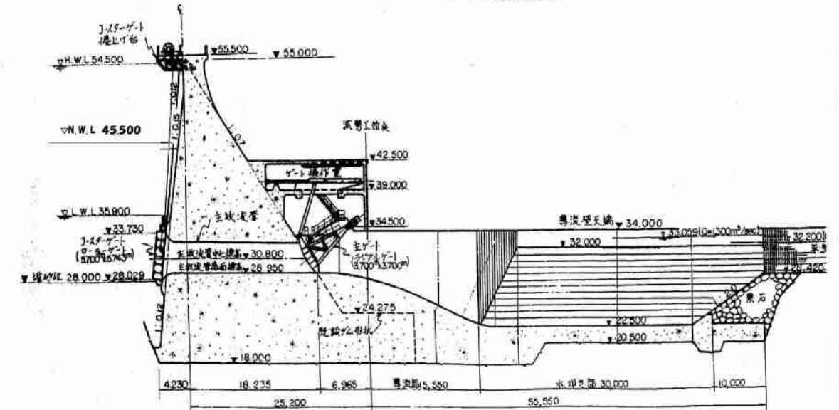
ダム縦断面図
