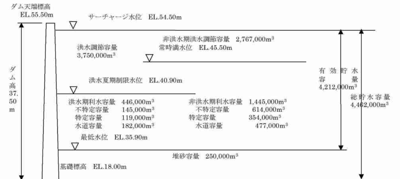
貯水池容量配分図 (再開発)
