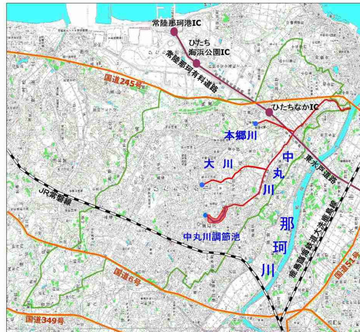
中丸川・本郷川・大川平面図
