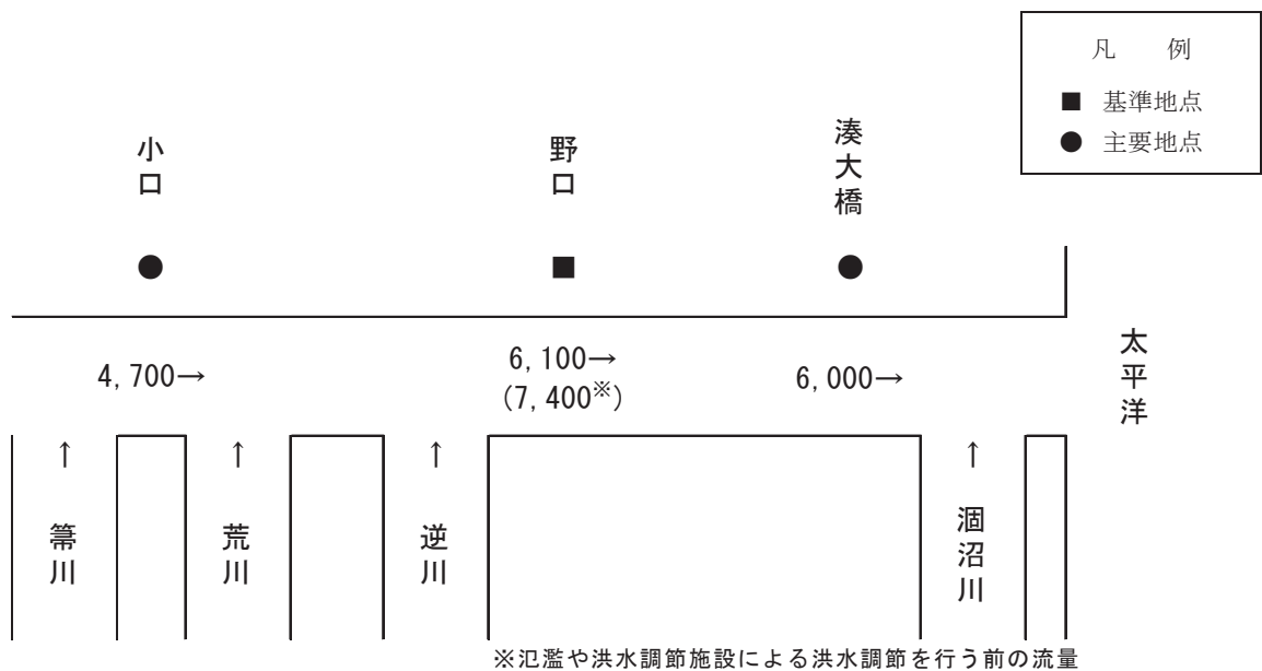
図 4-1 那珂川流量配分図 （単位：m³/s）
