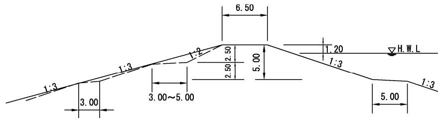
②小貝川 4.0～9.5k 縮尺1/500
