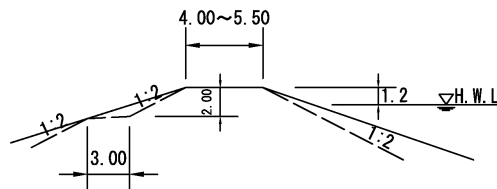
④大谷川 0.0～3.7k 縮尺1/500
