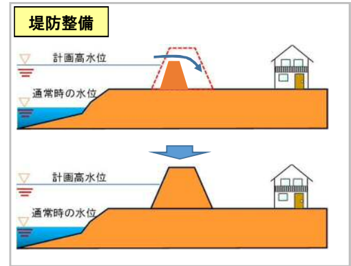
荒川 堤防整備事例(さいたま築堤)
