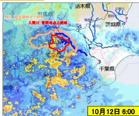
レーダー雨量図
