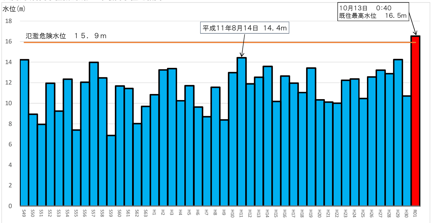
入間川(菅間水位観測所)の年最高水位比較図
