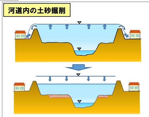
河道内の土砂掘削事例
