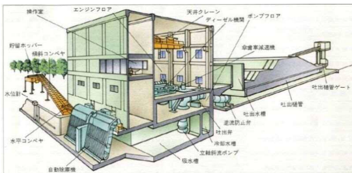
排水機場構成図
