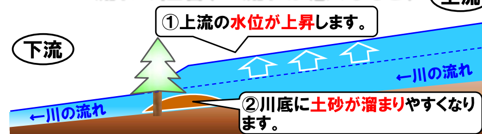
川の断面② 流れの阻害(=流れが悪くなると) (上流)
