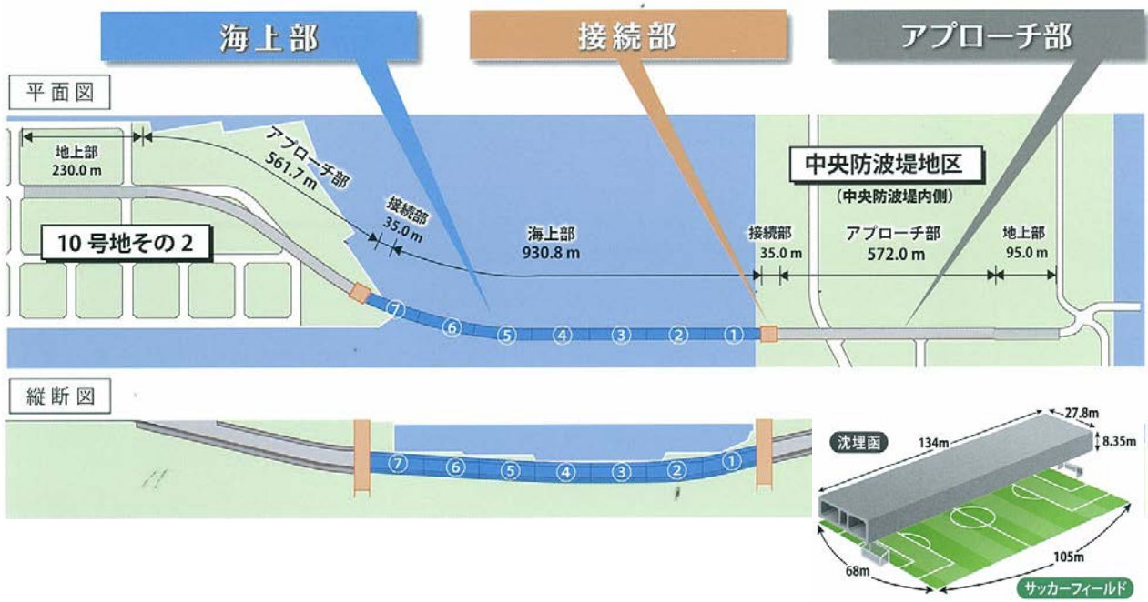
沈埋函の大きさ
