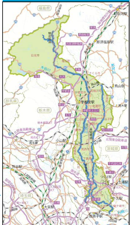
鬼怒川・小貝川の流域図
