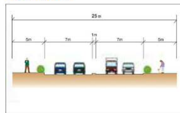
標準断面図
