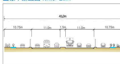
標準断面図（松原地区）
