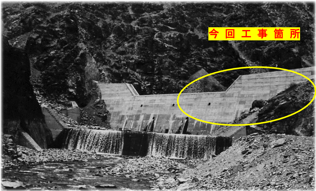
▲完成時の松木川一号砂防堰堤
