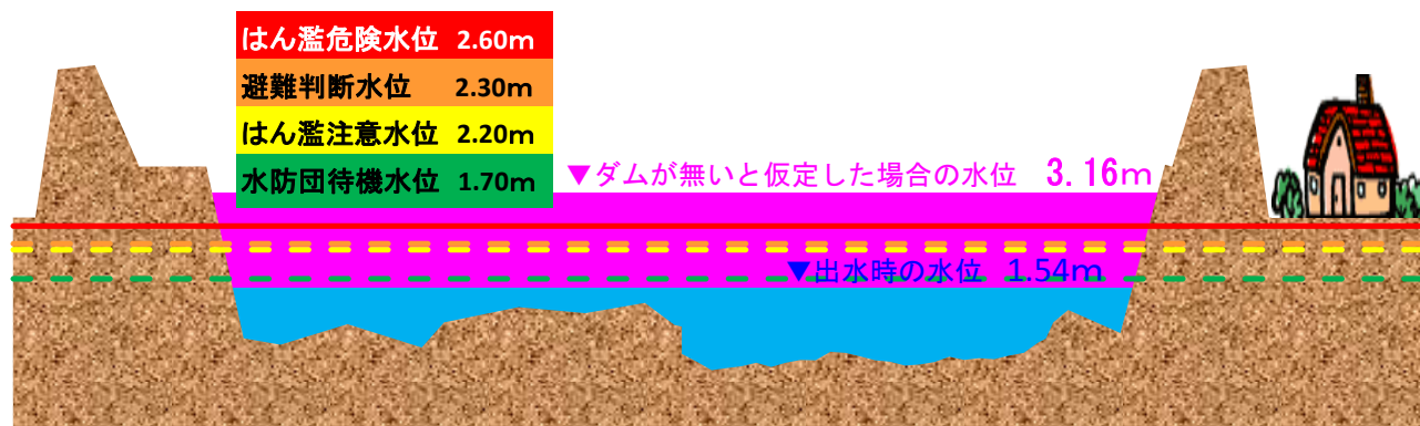
図2 宮ヶ瀬ダムにより想定される水位の低減（才戸橋地点）
