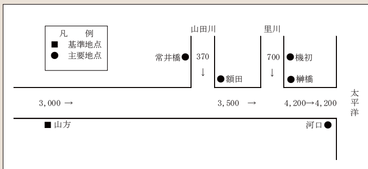
▲流量配分図
