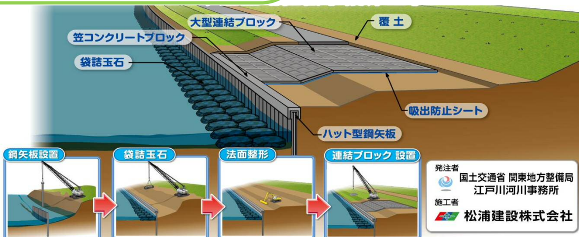
標準施工図
