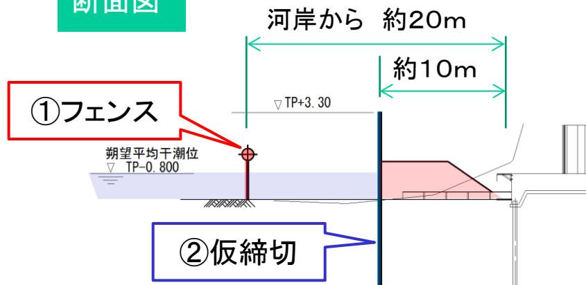
断面図
