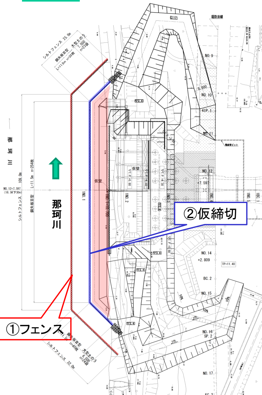
平面図
