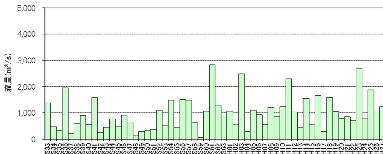
山方地点年最大流量の経年変化
