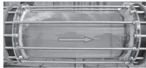
写真—2 滞留した空気が流される状況
