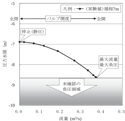
図—7 流量と配管頂部の圧力水頭 (レベル2)
