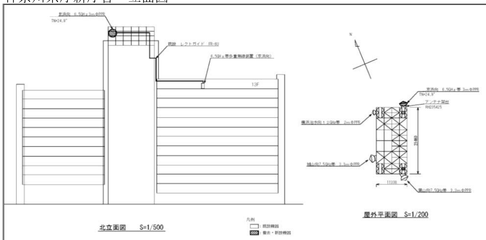
神奈川県庁新庁舎 立面図
