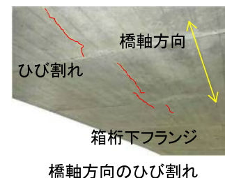
橋軸方向のひび割れ
