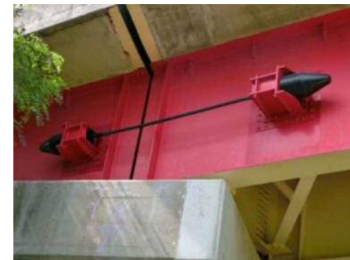
落橋防止構造P4
