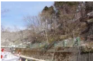
擁壁
