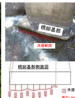
橋脚の洗掘
