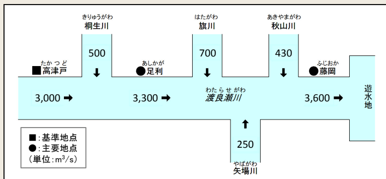
▲流量配分図
