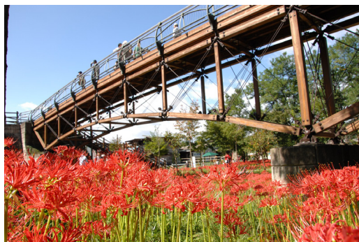
高麗郷の民族資料館と巾着田を結ぶ優美な「あいあい橋」は橋長91.2mで、木製トラス橋としては日本一の長さを誇ります
