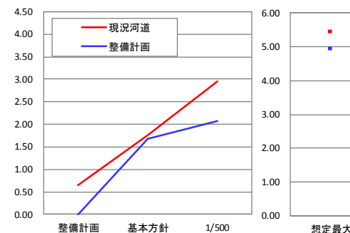
想定被害曲線【浸水面積(km 2 )】
