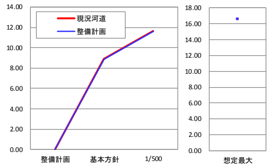
想定被害曲線【浸水面積(km 2 )】
