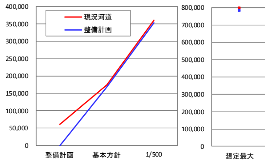
想定被害曲線【被害額(百万円)】
