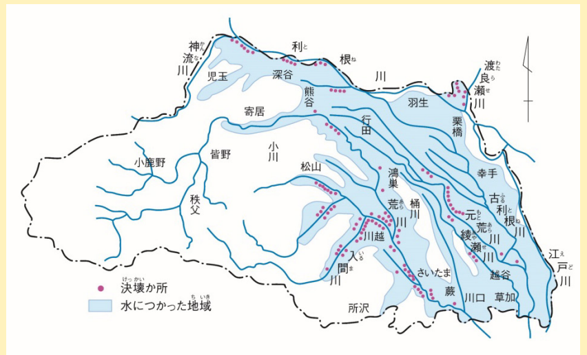
1910（明治43）年氾濫の図
