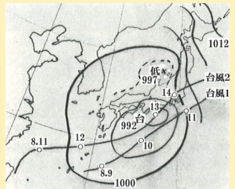
1910（明治43）年8月14日天気図
