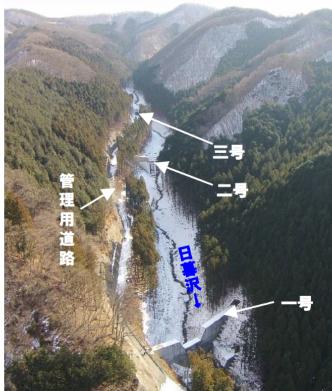
【砂防堰堤群全景】
