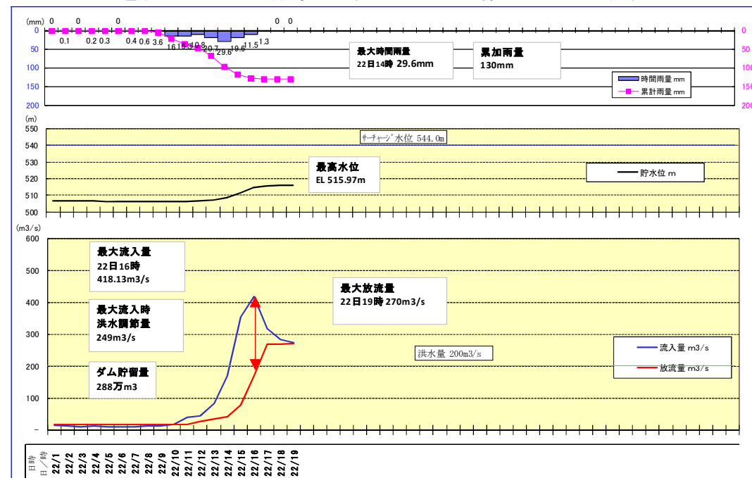
二瀬ダムの洪水調節効果(落合)
