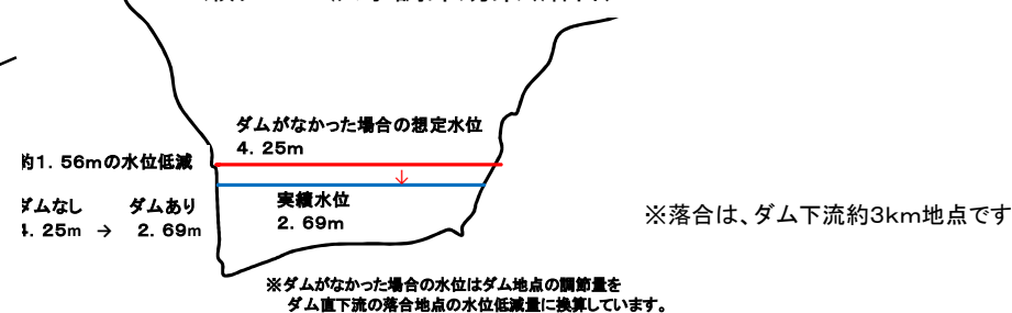
二瀬ダムの洪水調節効果(落合)
