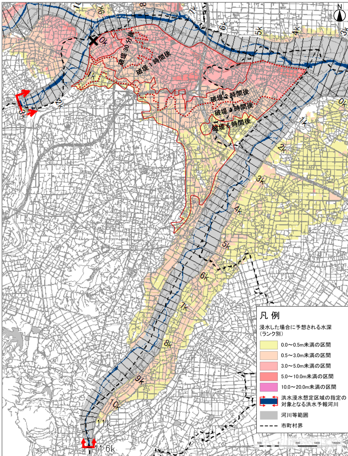
破堤箇所 鍬川 右岸 0.2k
