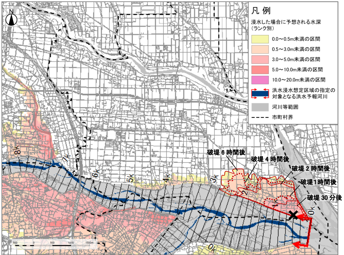
破堤箇所 烏川 左岸 0.4k
