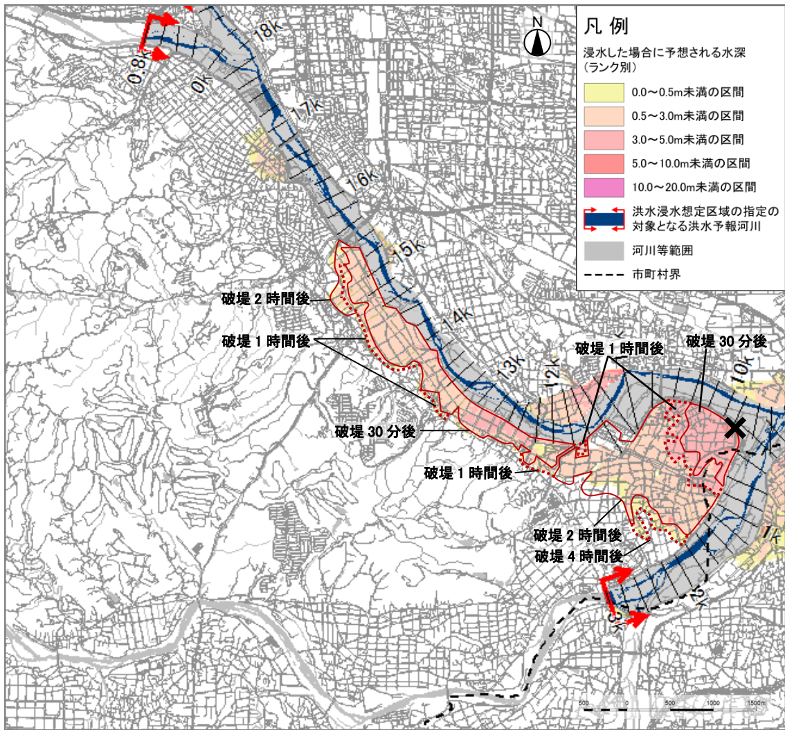
破堤箇所 烏川 右岸 9.8k
