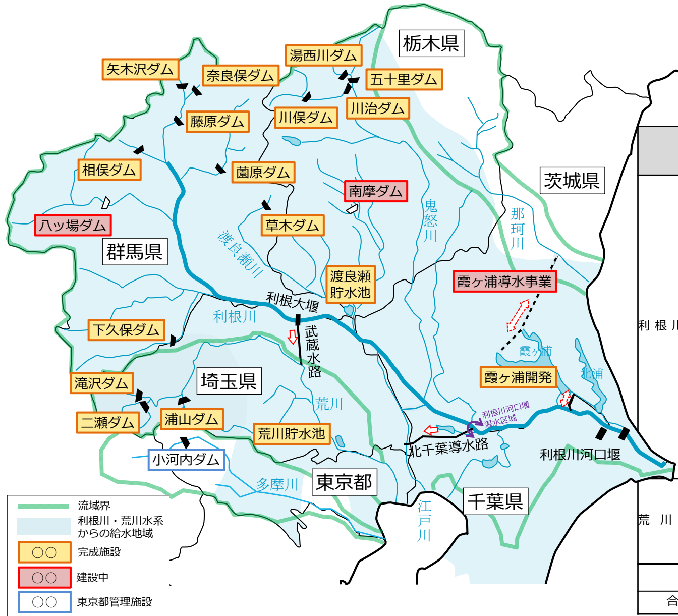
利根川・荒川水系の水資源開発施設
