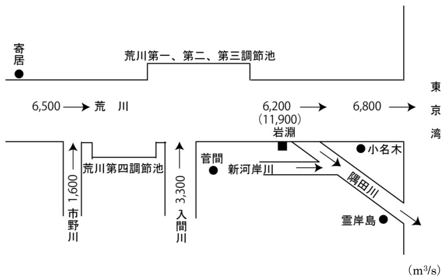
図 4-1 荒川整備計画流量図
