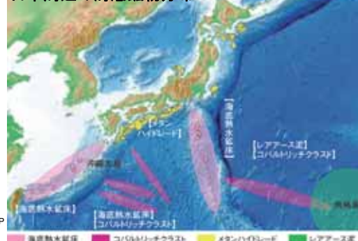
日本周辺の海底鉱物分布
