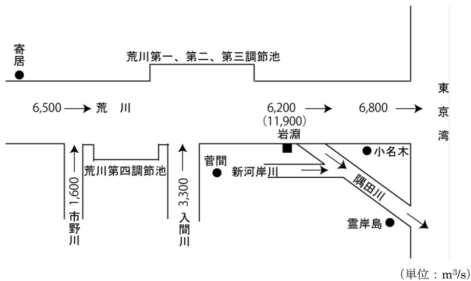
図 4-1 荒川整備計画流量図
