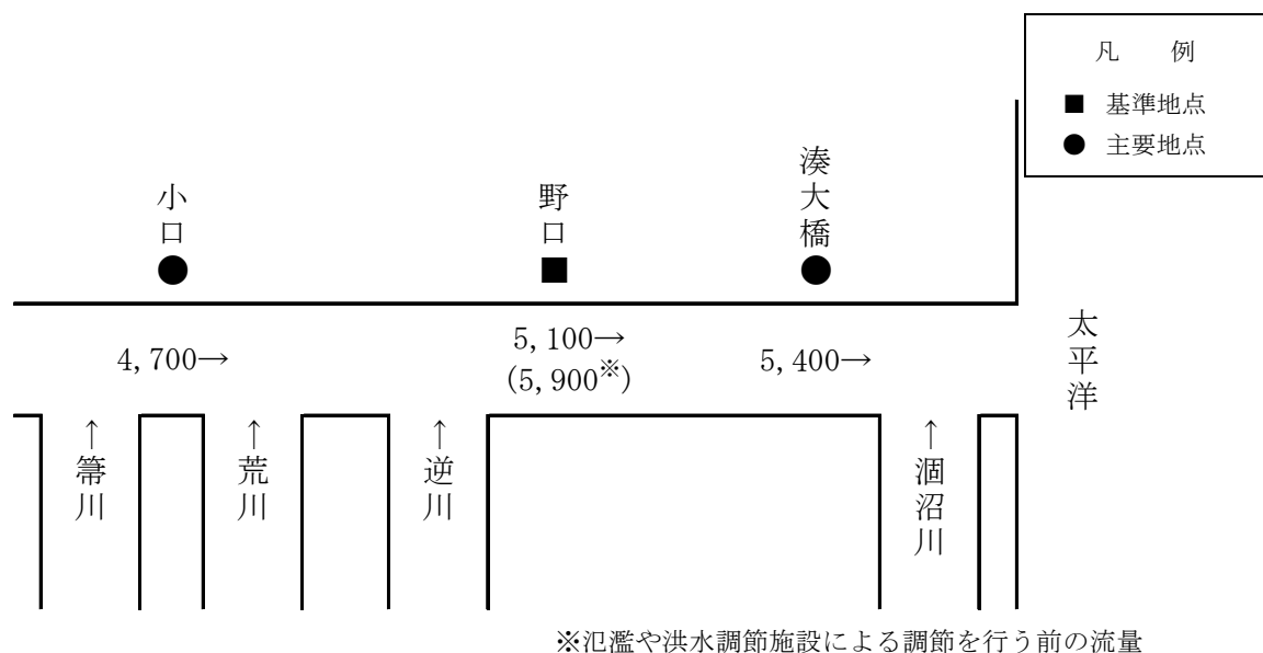
図 4-1 那珂川流量配分図 (単位: \text{m}^3/\text{s} )
