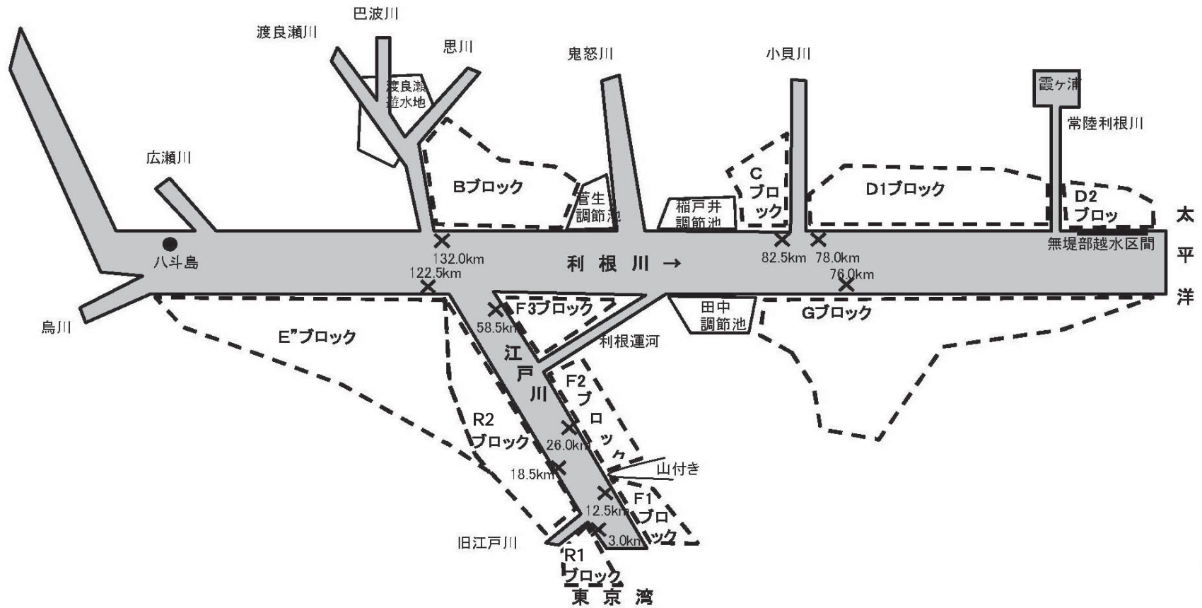
様式-1 氾濫ブロック分割図(利根川、江戸川)
