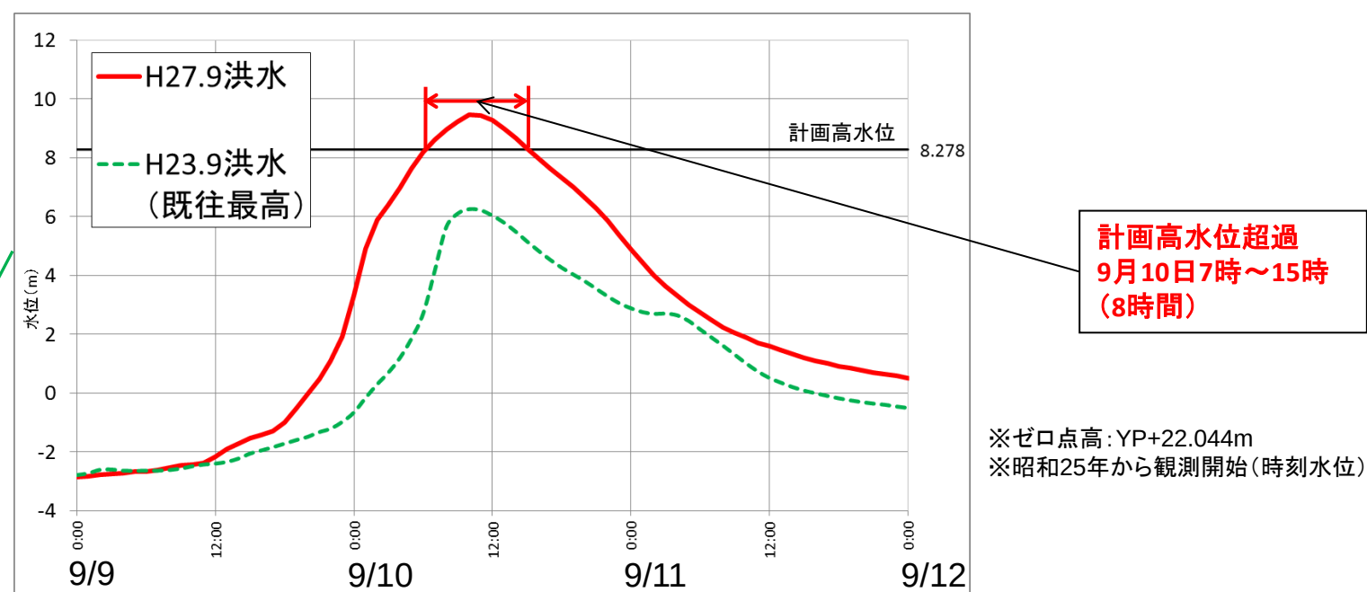
鬼怒川水海道地点
