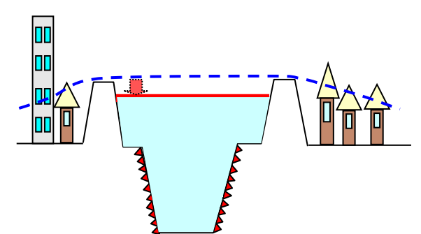
拡幅・築堤による改良工事
