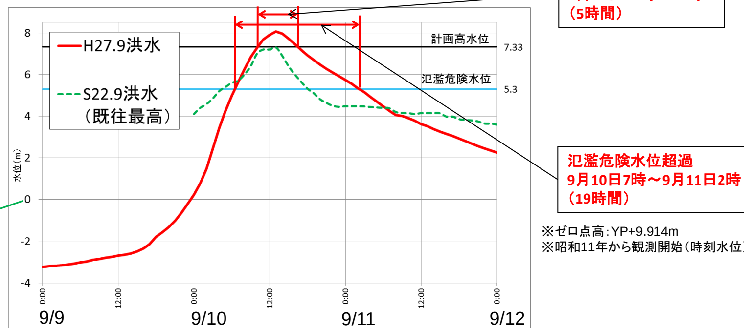
鬼怒川水海道地点
