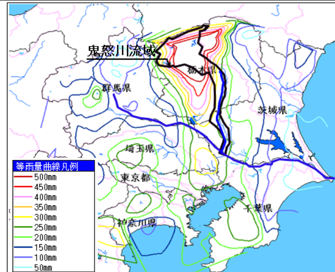
等雨量線図(8日~10日累加雨量)
