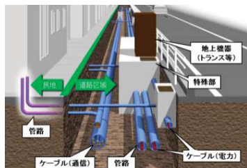
【電線共同溝方式による無電柱化】
